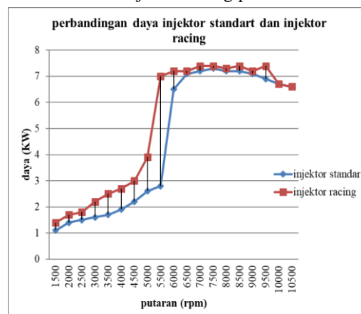
Gambar 1 Grafik hasil perbandingan daya injektor standart dan injektor racing
