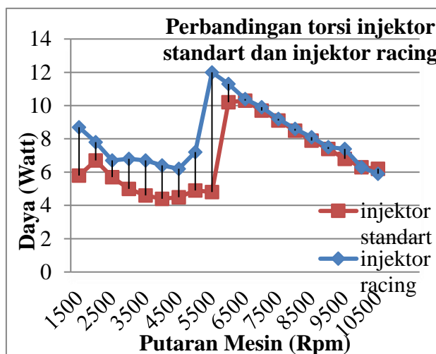
Gambar 2 Grafik Hasil perbandingan torsi injektor standart dan injektor racing.
