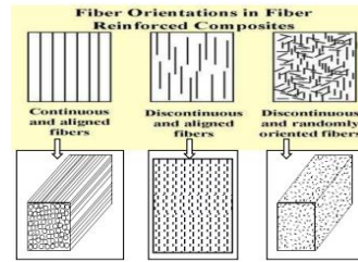
Gambar 4. Jenis serat fiber
