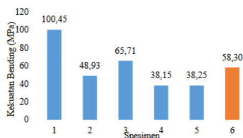
Gambar 1. Grafik Hubungan Campuran Resin dan Serat Buah Pinang Terhadap Kekuatan Bending
