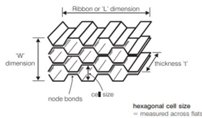
Gambar 7. Struktur Honeycomb
