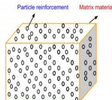
Gambar 3. Bentuk partikel
