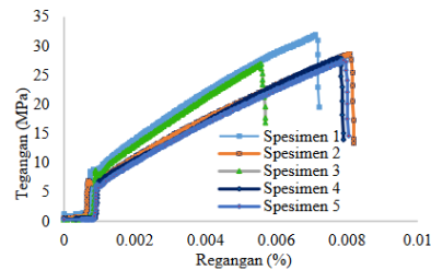
Gambar 2. Grafik Tegangan-Regangan Resin dan Serat Buah Pinang
